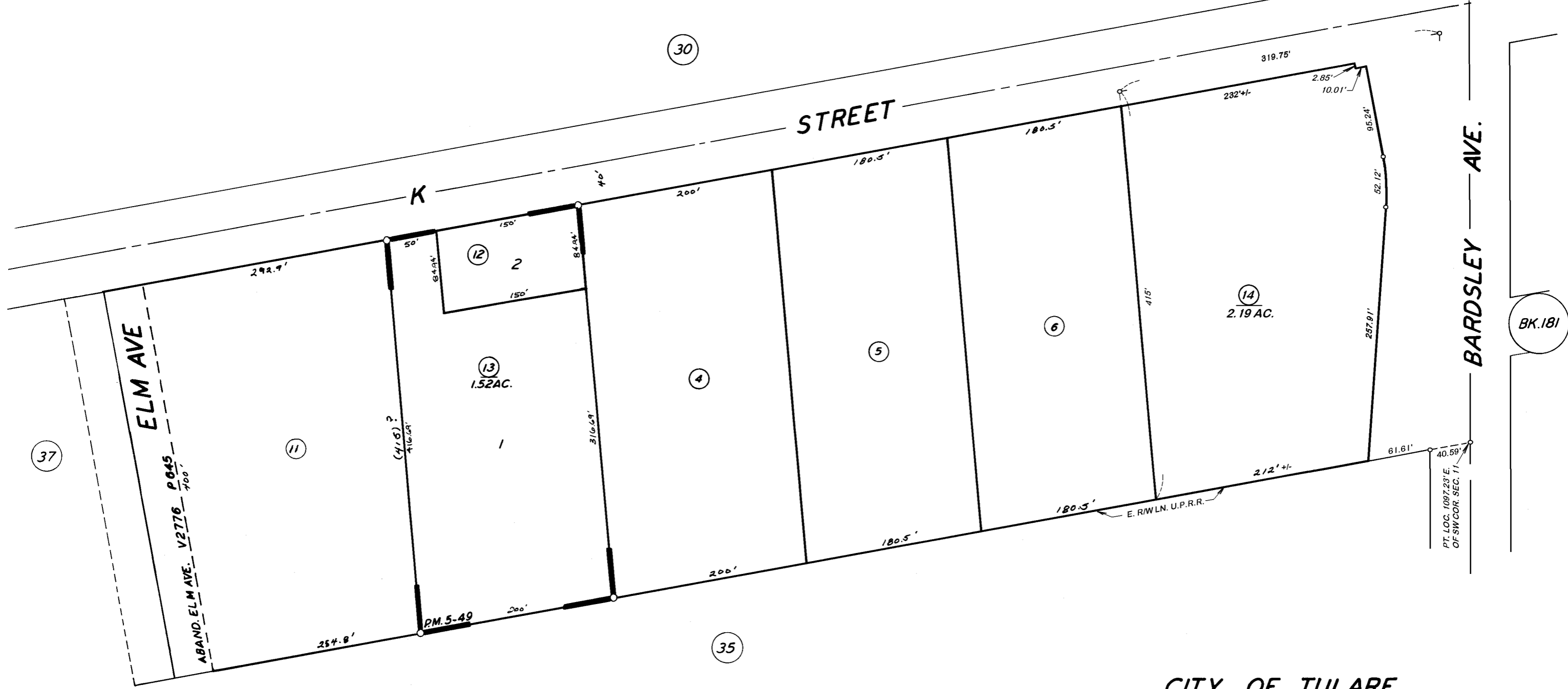
PARCEL MAP 449, P.M.5-49
